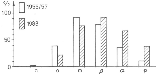
Abb. 3: Hemerobiety-Spektren 1956/57 und 1988.
