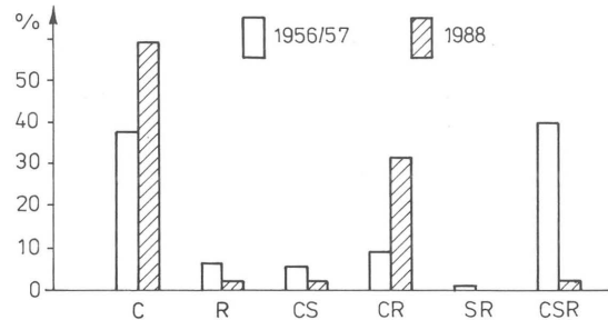
Abb. 4: Strategietypen-Spektren 1956/57 und 1988.
