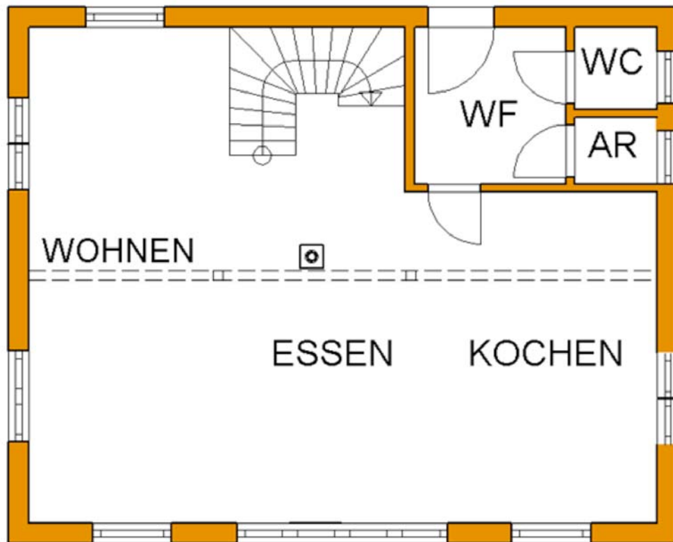
Grundriss EG
